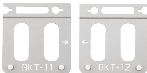
BKT11 & BKT12 SUPPORT POUR TRU-POINT
